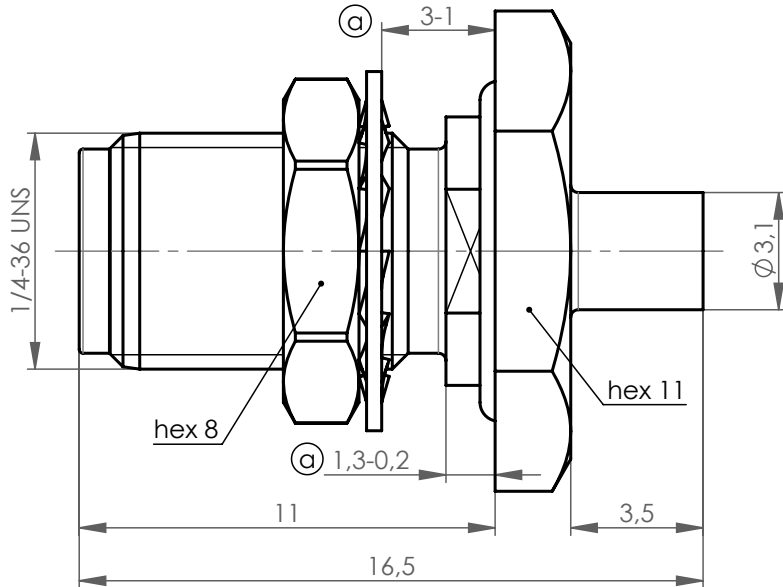
mounting dimensions / Einbaumaße Z027
