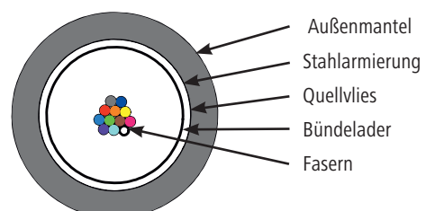
A-DQ(ZN)(SR)B2Y 1xX
