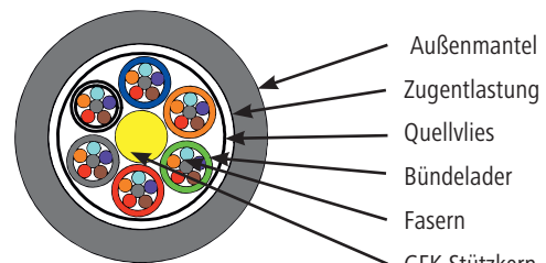
A-DQ(ZN)B2Y 4x12
